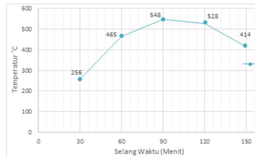
Gambar 9. Temperatur pembakaran briket pakis hutan
