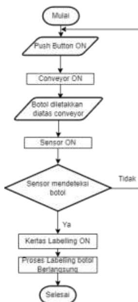
Gambar. 8 Flowchart Cara Kerja Alat
