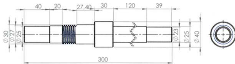
Gambar 4. Poros pencacah
