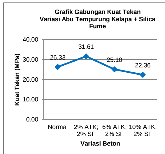
Gambar 6. Grafik pengujian kuat tekan variasi campuran
