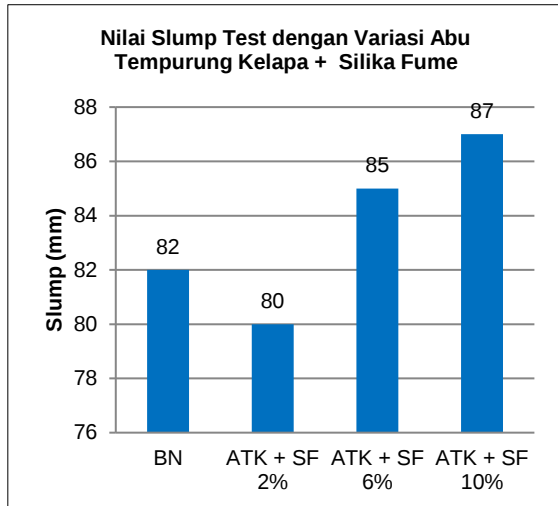
Gambar 5. Grafik variasi campuran dengan nilai slump
